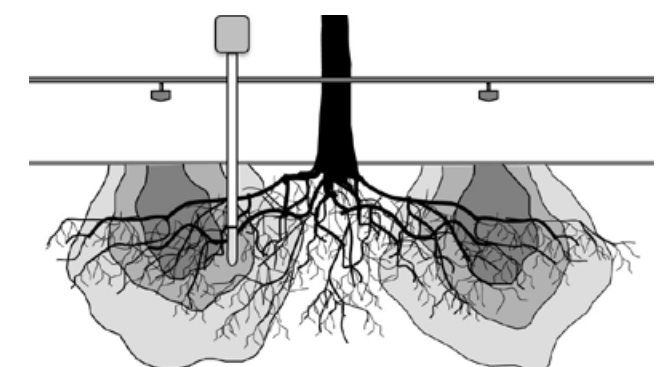
Abb.2: Schematische Darstellung der Bodenfeuchtemessung mit einem Tensiometer
